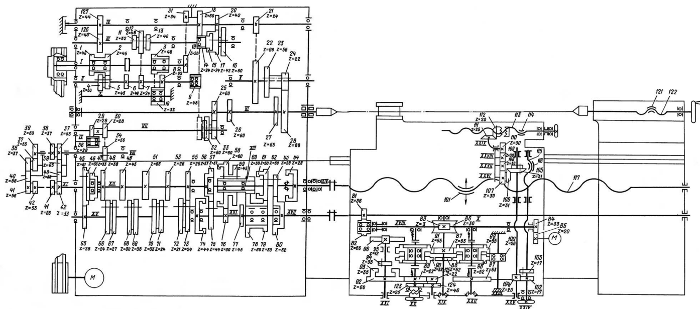
Рис. 4. Схема кинематическая
